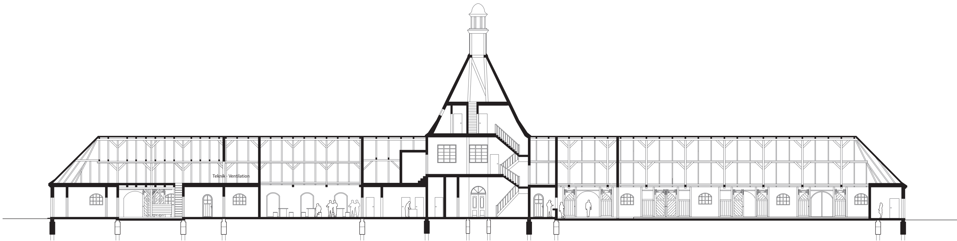
LÆNGDESNIT 1:250
