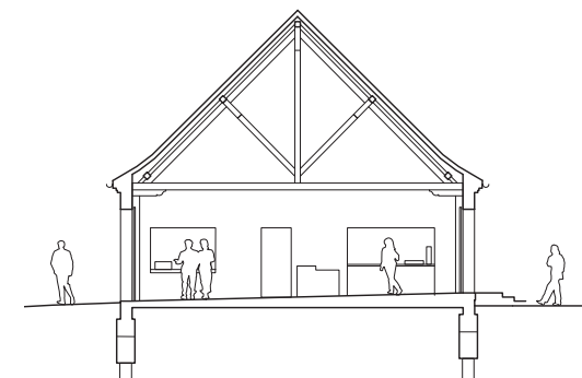
SNIT BB i Besøgscenter 1:250
