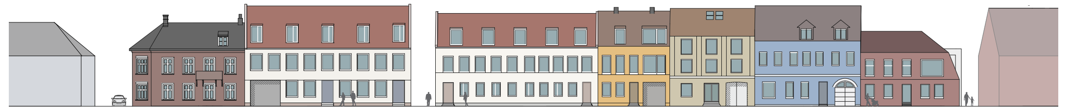
Havregade - Opstalt fra Kongenstøfte til Tolderensstræde - fremtidige forhold - 1:500
