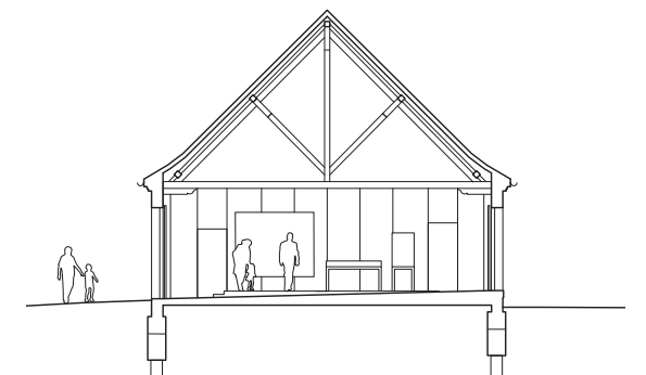
SNIT CC i Udstillingssal 1:250
