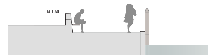
Højvandsikring langs Havnepromenaden - fremtidige forhold 1:100
